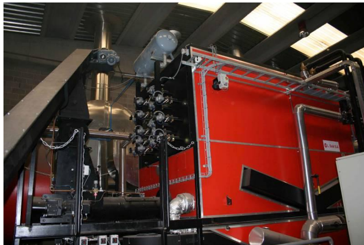
Fig. 3.5. Vista del local tècnic d'una instal·lació de calefacció de barri de 2 MW amb biomassa, a Molins de Rei.
