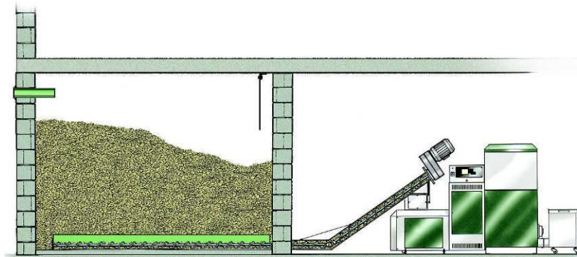
Fig. 5.7 El vis sens fi que surt de la sitja, puja per a carregar la tremuja adjunta a la caldera domèstica, de la qual s'abasteix el cremador.
