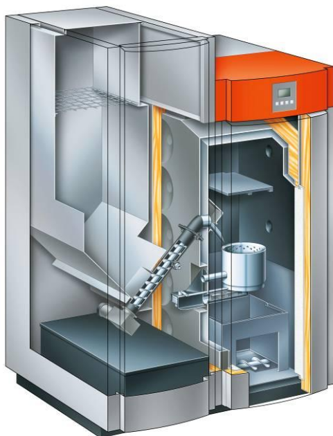
Fig. 5.6 Vista interior d'una caldera domèstica on es pot apreciar la tremuja adossada, amb el vis sens fi a la part baixa que alimenta el gresol.
