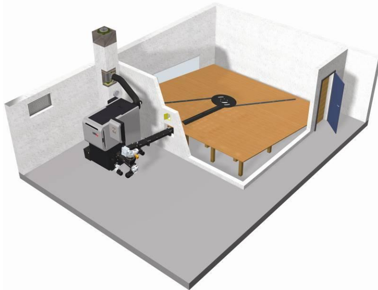
Fig. 5.10 Imatge d'una instal·lació de caldera de biomassa domèstica amb ballesta remenadora i accés protegit a la sitja.
