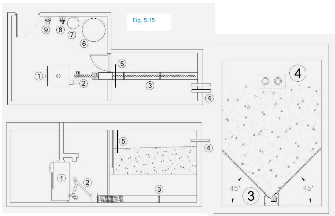
Fig. 5.15 Local tècnic de biomassa de 50kW, en què: 1- Caldera de biomassa; 2- Vis sens fi d'alimentació sitja-caldera; 3- Ramps de sitja i vis sens fi; 4- Guillemines de càrrega; 5- Lona amortidora; 6- Dipòsit inercial de 1.000 litres; 7- Dipòsit d'ACS; 8- Sistema de bombament per a la distribució de la calefacció; 9- Sistema de bombament per a la distribució de l'ACS.
