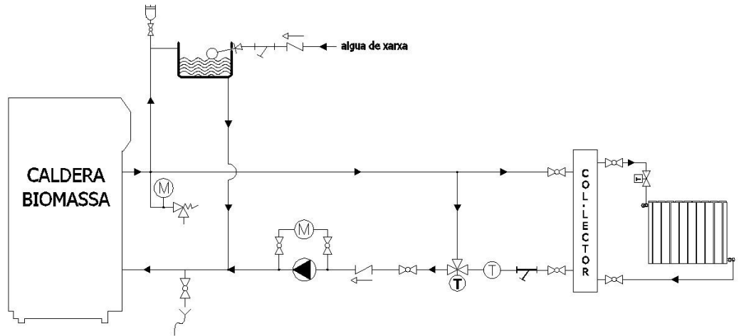
Fig. 7.2. Esquema bàsic d'instal·lació en circuit obert. Es pot dotar la instal·lació d'un bescanviador previ a la distribució de radiadors, en cas de dificultats amb les alçades relatives o instal·lació de terra radiant.
